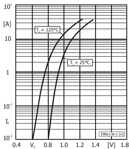
Forward characteristics (typical values) Durchlasskennlinien (typische Werte)
